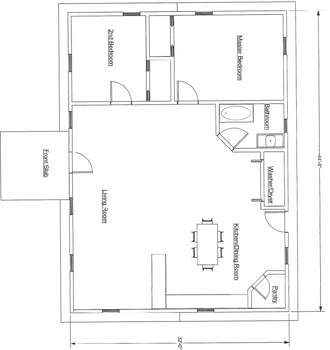
1 House #1 Scale: 1/8" = 1'-0"
